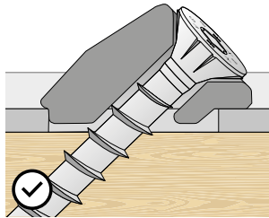
VGU inclined washer
