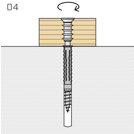
通过拧紧螺钉而固定板条，使头部与木构件齐平。
