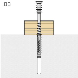
定位 DRT 螺钉。
