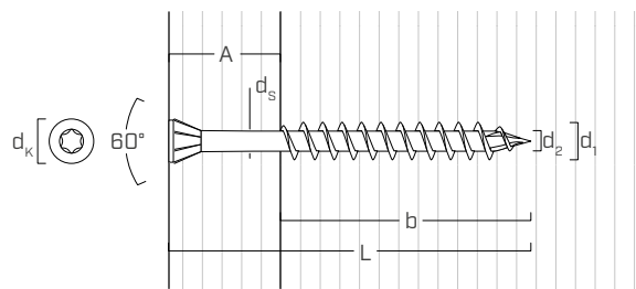
SHSAS Ø3,5
