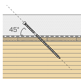
Colocación a 45° con lámina fonoaislante.
