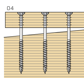
Nastavenie ostatných skrutiek rovnakým spôsobom pre vyrovnanie konštrukcie.
