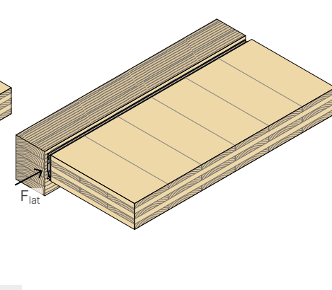
gerenda | CLT földém
